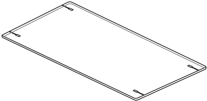
MENSOLA RETTANGOLARE accessori esclusi materiale: plexiglass trasparente 6mm misure (mm): 265x410x6h cod.art: MSRS
