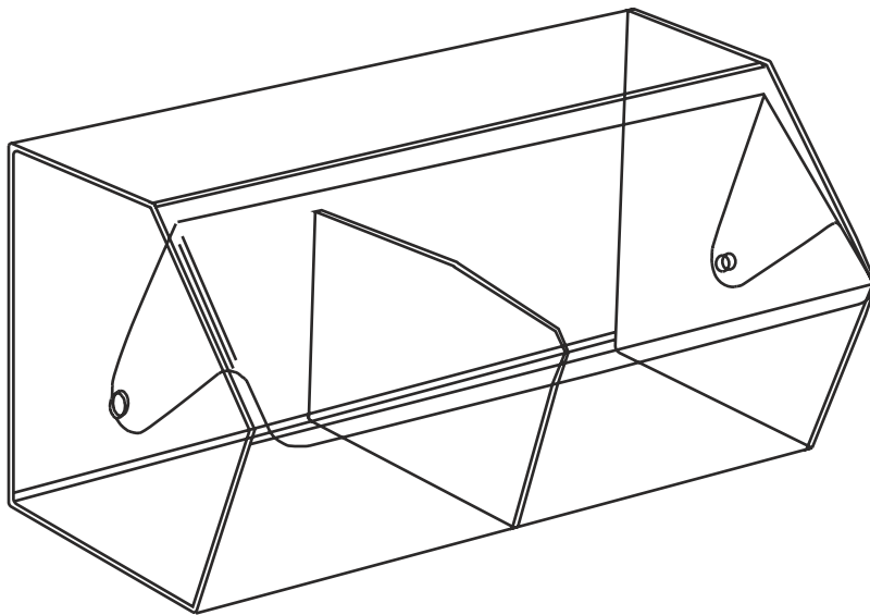
PORTACIALDE DOPPIO materiale: plexiglass trasparente 3mm misure (mm): 300x200x155h cod.art: PCDD
