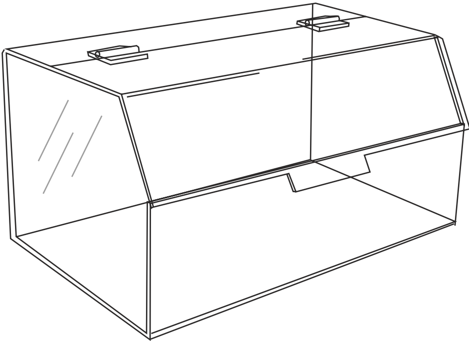
CASSETTA BRIOCHE materiale: plexiglass trasparente 4mm misure (mm): 435x255x275h cod.art: CBR1
