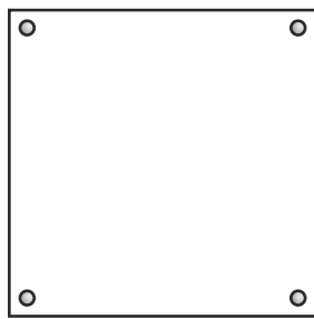
TARGA QUADRATA materiale: plexiglass trasparente 8mm misure (mm): 430x8x430h cod.art: TAPO-Q
