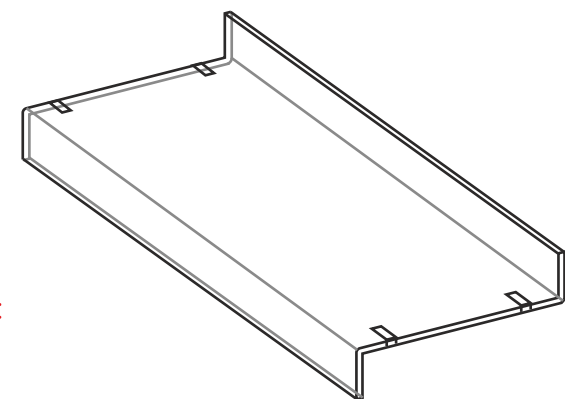
MENSOLA "L" accessori esclusi materiale: plexiglass trasparente 6mm misure (mm): 210x280x86h cod.art: MSZS
