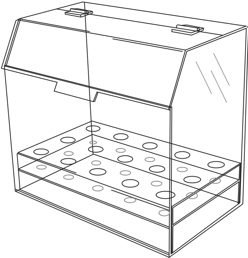
CASSETTA PORTACONI materiale: plexiglass trasparente 4mm misure (mm): 410x250x380h cod.art: CTP1
