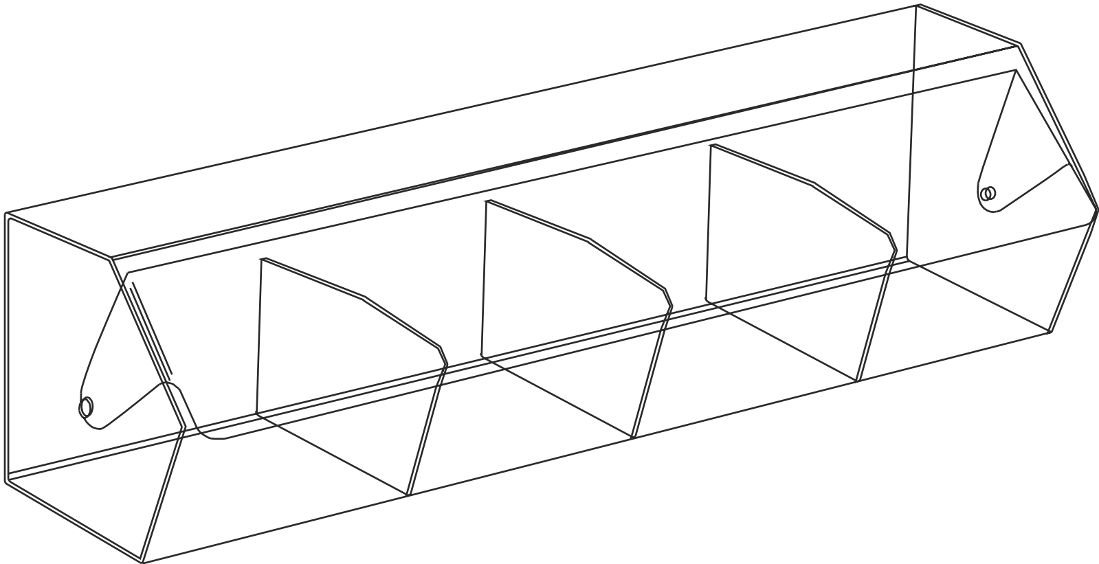
PORTACIALDE QUADRUPLO materiale: plexiglass trasparente 3mm misure (mm): 450x200x155h cod.art: PCDQ
