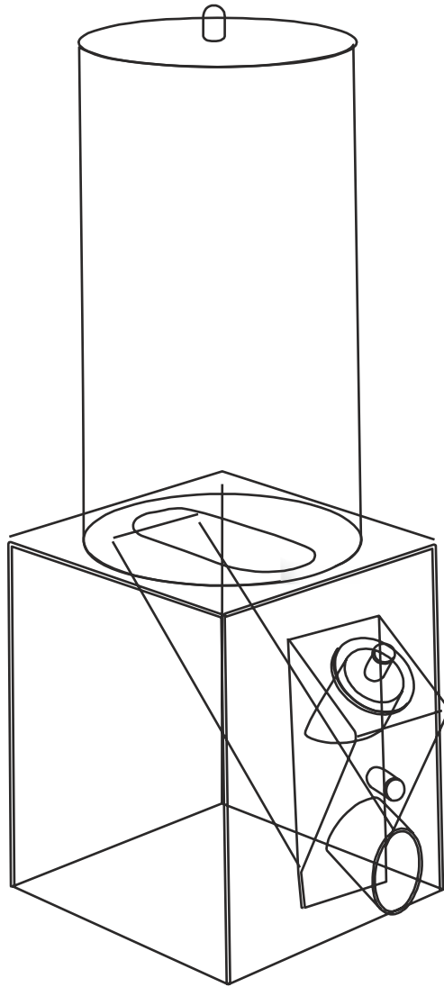
SILOS PER CAFFÈ materiale: plexiglass trasparente 5mm misure (mm): 300x220x620h diametro (mm): 200 capacità: 3,3kg cod.art: 701-S4
