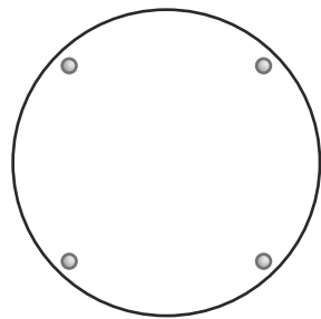
TARGA CIRCOLARE materiale: plexiglass trasparente 8mm misure (mm): 430x8x430h cod.art: TAPO-C
