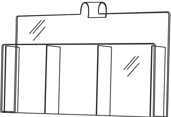
TASCA TRIPLO DEPLIANT materiale: plexiglass trasparente 3mm misure (mm): 360x80x235h cod.art: PX120TD
