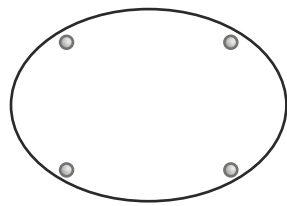
TARGA OVALE materiale: plexiglass trasparente 8mm misure (mm): 430x8x300h cod.art: TAPO-O
