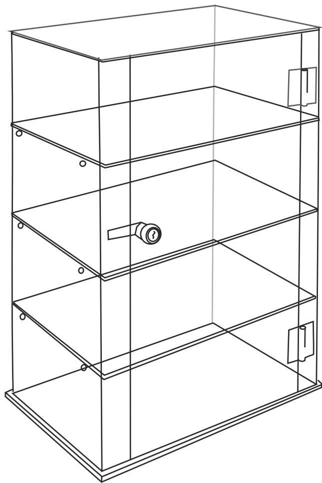
ESPOSITORE MIRÒ chiusura a chiave materiale: plexiglass trasparente 4mm misure (mm): 305x210x560h cod.art: ESMI55
