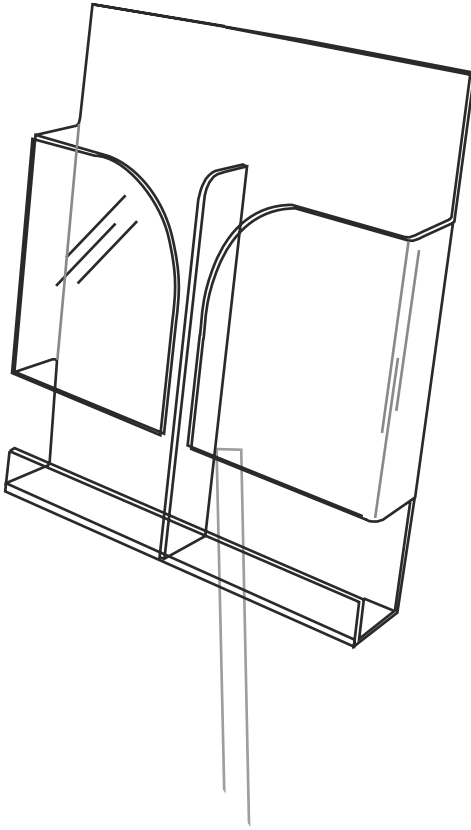
TASCA DOPPIO DEPLIANT materiale: plexiglass trasparente 3mm misure (mm): 220x100x270h cod.art: PNT90DD
