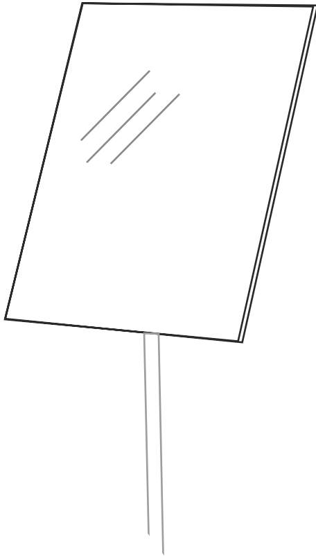
SUPPORTO A4 materiale: plexiglass trasparente 3mm misure (mm): 210x50x300h cod.art: PNT90A4
