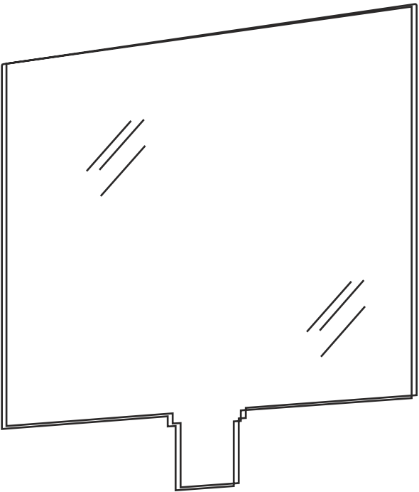
SUPPORTO A3 materiale: plexiglass trasparente 3mm misure (mm): 420x370h cod.art: PX120A3
