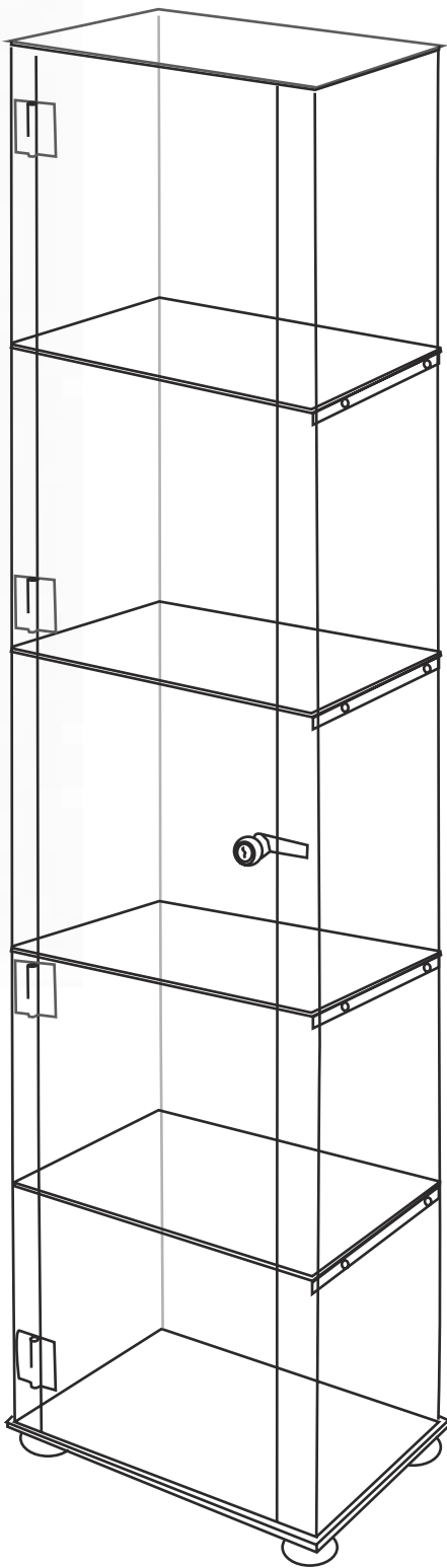
VETRINA MIRÒ chiusura a chiave e ruote pivotanti materiale struttura: plexiglass trasparente 4mm materiale mensole: plexiglass colorato 3mm misure (mm): 350x350x1500h cod.art: VTRM150
