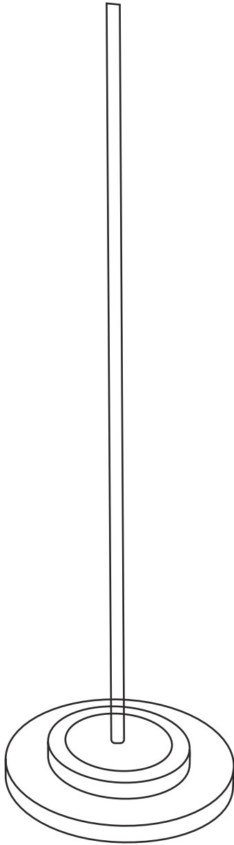
PIANTANINA STRUTTURA materiale: plexiglass trasparente 15mm misure (mm): 215x245x840h cod.art: PNT90
