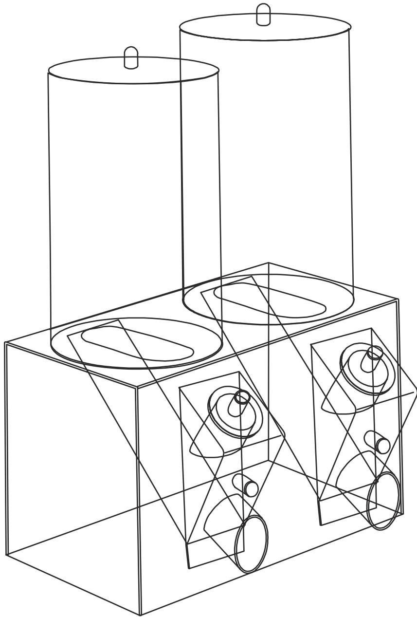
SILOS PER CAFFÈ DOPPIO materiale: plexiglass trasparente 5mm misure (mm): 300x430x620h diametro (mm): 200 capacità: 6,6kg cod.art: 701-D8
