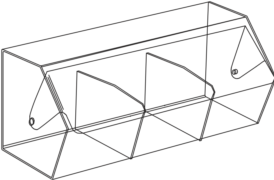
PORTACIALDE TRIPLO materiale: plexiglass trasparente 3mm misure (mm): 340x200x155h cod.art: PCDT
